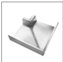
Binnenhoekstuk voor bakgoot, 90 graden
