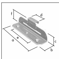
RHEINZINK Clipfix RVS schuifklang standaard
