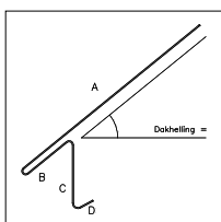
Druiprandprofiel
