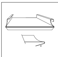
Felsbaan, uitgestanst/omgezet zink 0,80 mm / koper 0,70 mm
