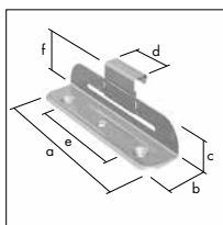
RHEINZINK Clipfix RVS schuifklang hoog
