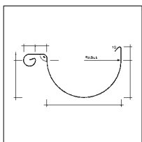
Maatmastgoten, standaardlengte 3 m met KOMO-keur
