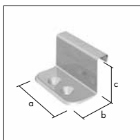
RHEINZINK Clipfix RVS vaste klang standaard
